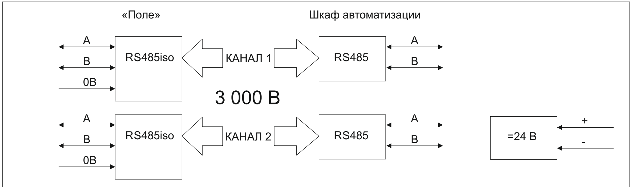
Функциональная схема прибора РИ4852
